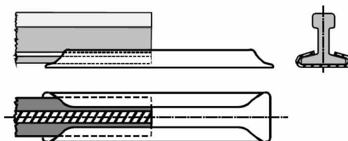
Slika 2. Spjalica.
