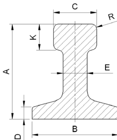
Slika 1. Oblik tračnice
